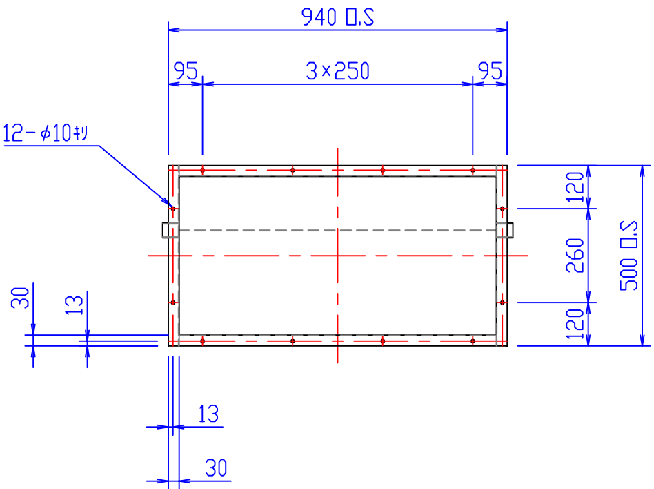
A-A矢視；本体固定用ボルト位置
