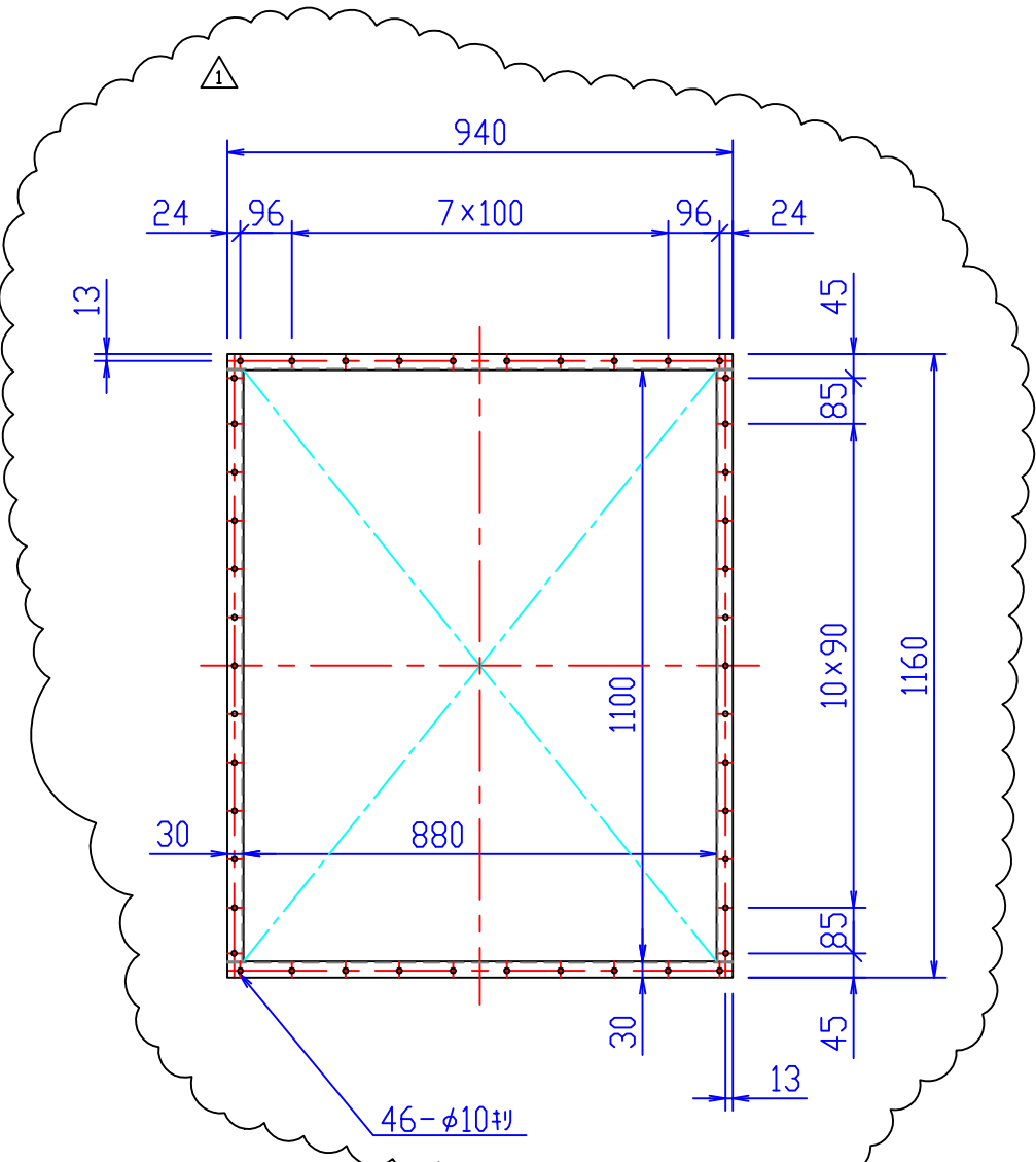
フランジ寸法図
