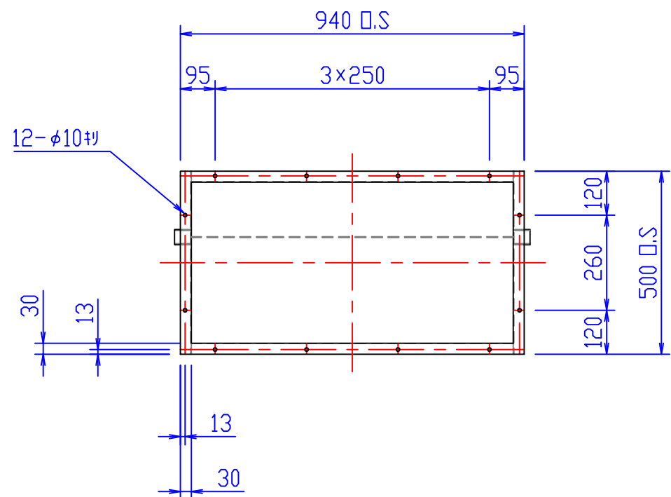
A-A矢視：本体固定用ボルト位置
