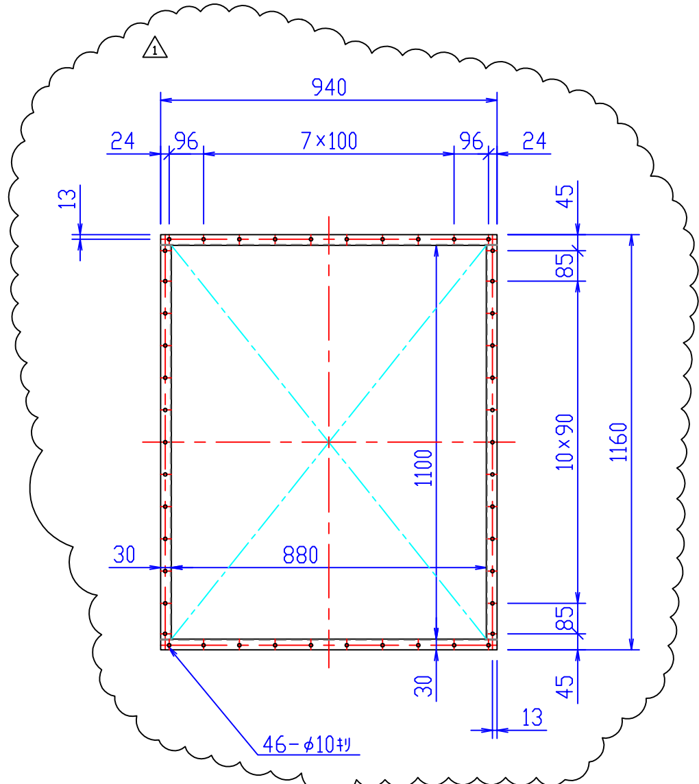
フランジ寸法図
