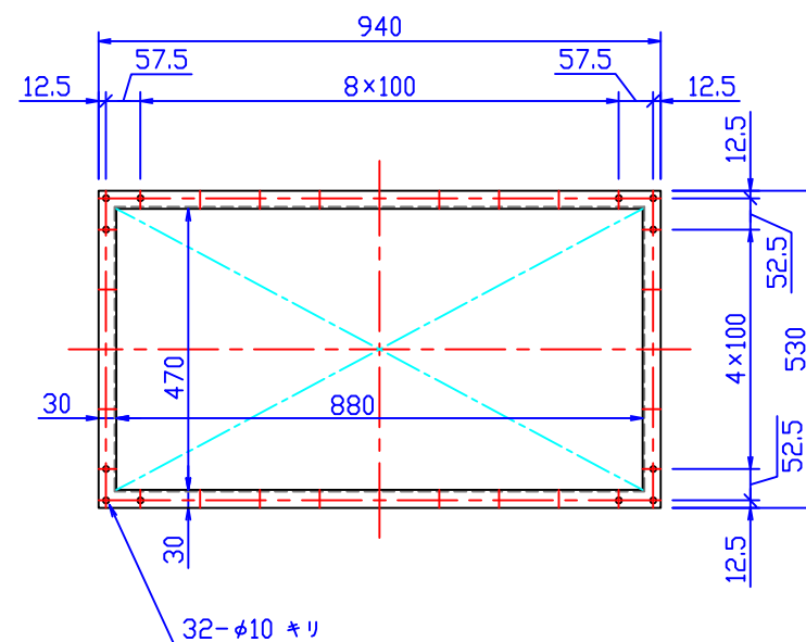
フランジ寸法
