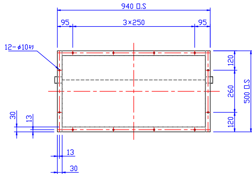
A-A矢視；本体固定用ボルト位置
