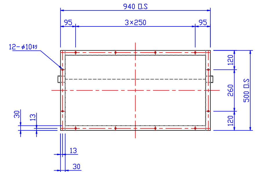
A-A矢視；本体固定用ボルト位置
