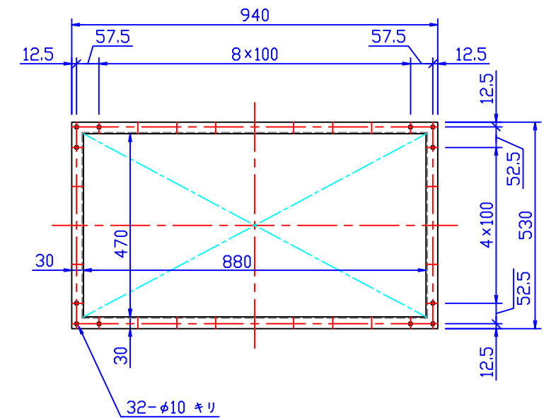
フランジ寸法
