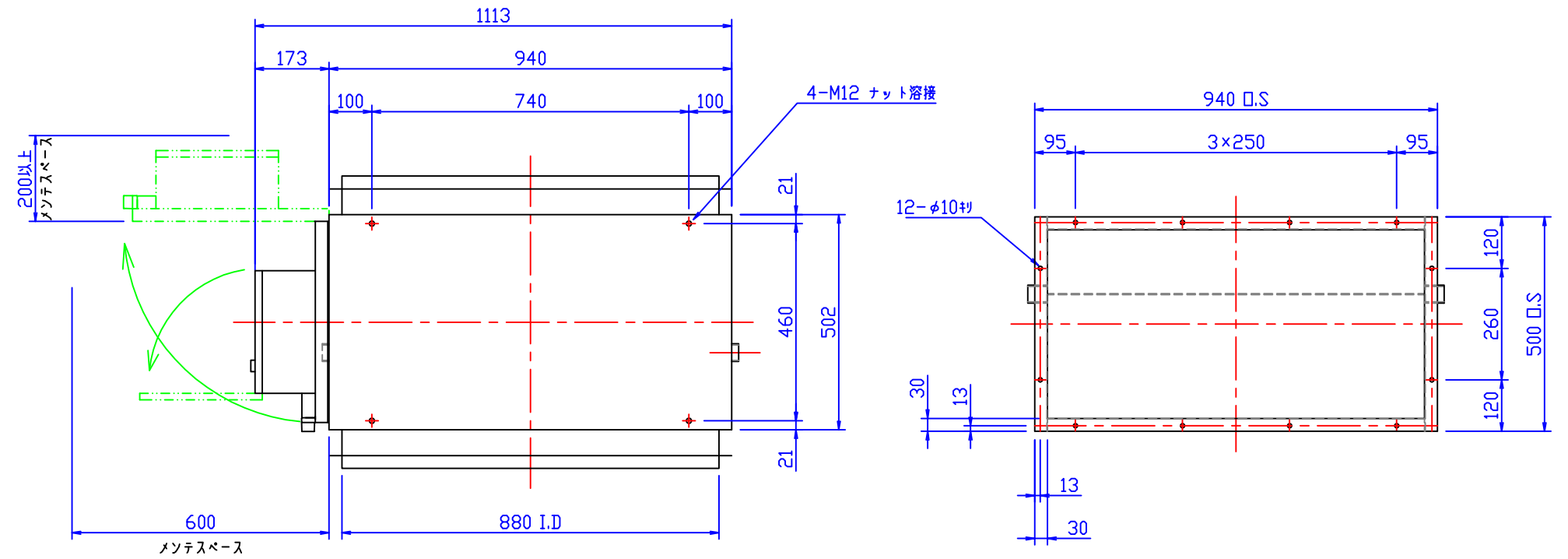
A-A矢視；本体固定用ボルト位置
