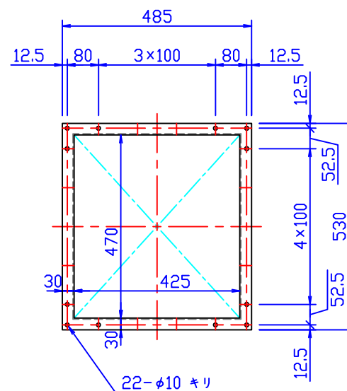
フランジ寸法
