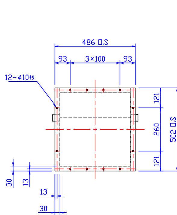
A-A矢視；本体固定用ボルト位置
