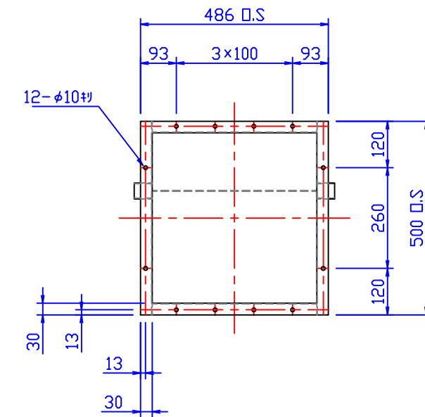
A-A矢視；本体固定用ボルト位置
