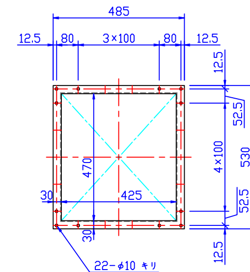
フレンジ寸法
