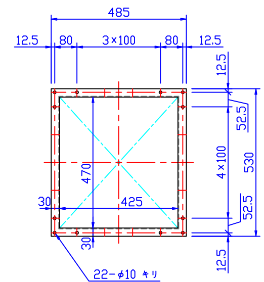
フランジ寸法
