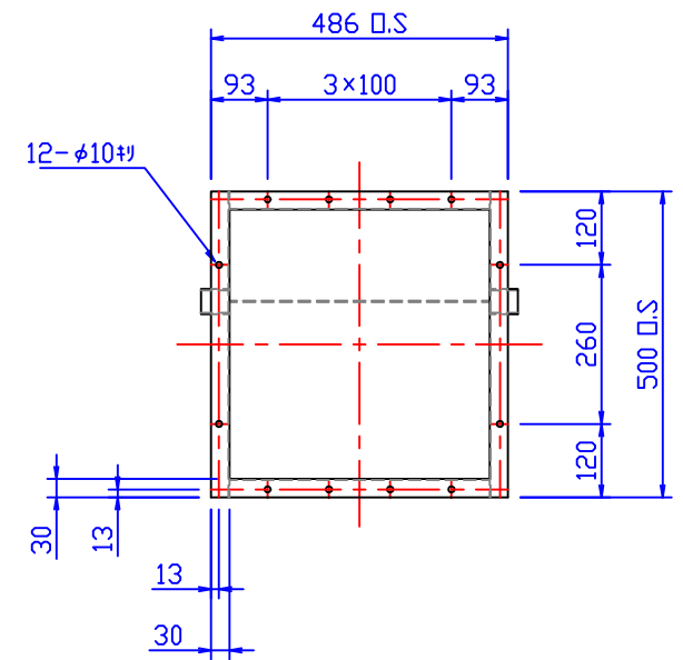
A-A矢視；本体固定用ボルト位置
